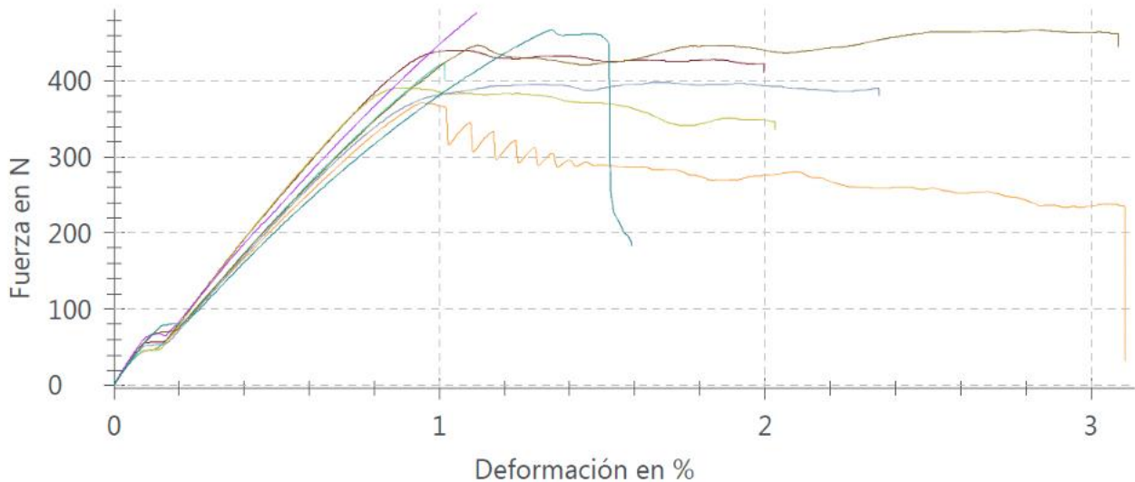
Figura 8. Ensayos de tracción triplicados formulación A, B y C. Las pruebas demuestran las diferentes resistencias de los materiales.
