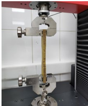
FIGURA 7. Ensayos de tracción. Las pruebas confirman la estabilidad dimensional y la resistencia del material frente a condiciones de tracción.
